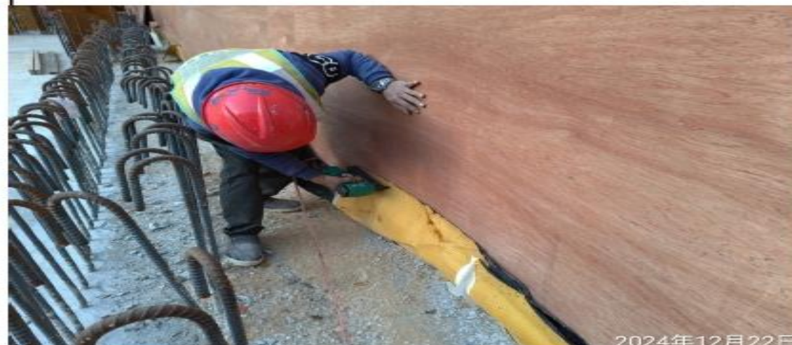
說明：B2FL外牆防水膜補強。
